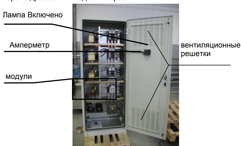
Рис.1 Внешний вид установок серии ВАРНЕТ-НФ.
