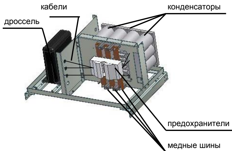
Рис.2 Внешний вид модулей для установок серии ВАРНЕТ-НФ.
