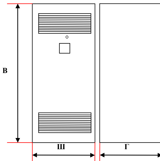
Рис.8 Габаритный чертеж установок ВАРНЕТ-НФ.
