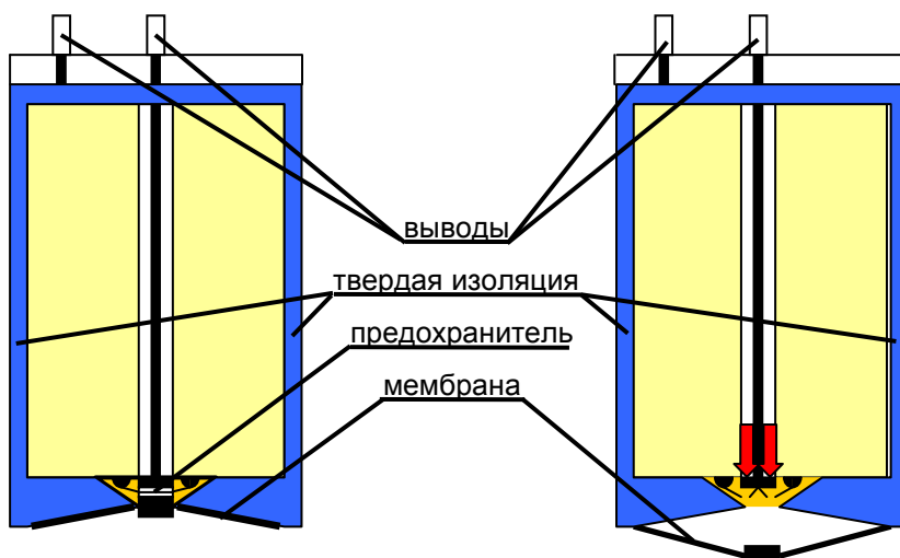
а) до срабатывания б) после срабатывания Рис.4 Принцип действия устройства защиты от превышения давления.
